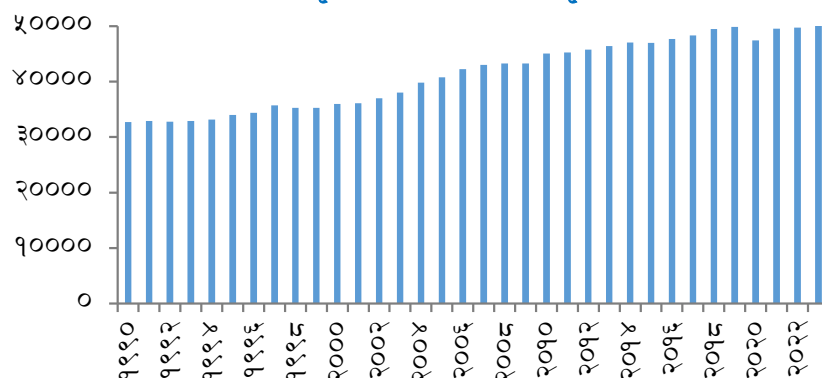
चार्ट १४(क): विश्वको हरितगृह ग्यास उत्सर्जनको प्रवृत्ति (दशलाख टन CO 2 )
